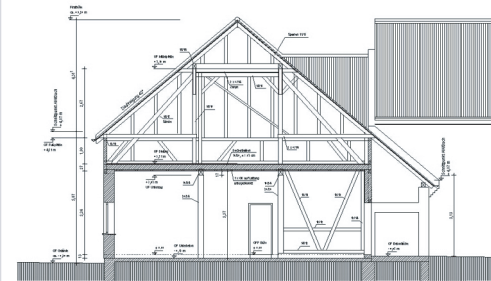
Gebäudequerschnitt A-A
